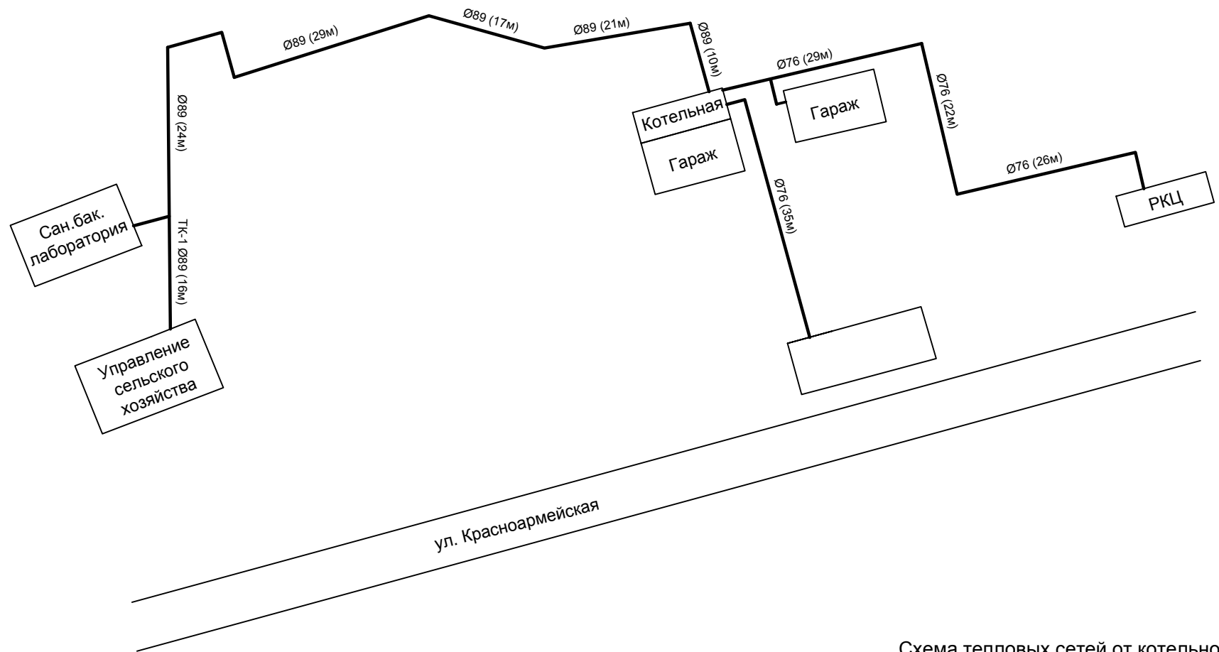
Схема тепловых сетей от котельной, расположенной по ул. Красноармейская
